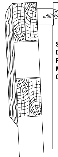
SECCIÓN TRANSVERSAL DEL SISTEMA DE PROTECCIÓN DEL MUELLE FRONTAL CON LA SERIE 700
