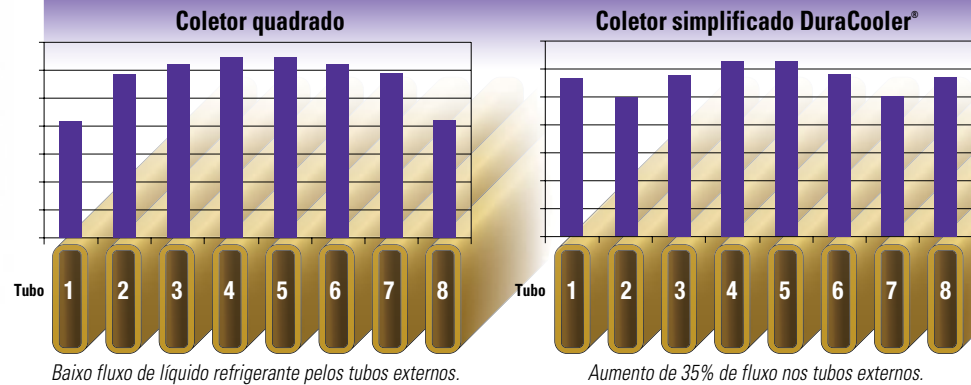
Baixo fluxo de líquido refrigerante pelos tubos externos.
